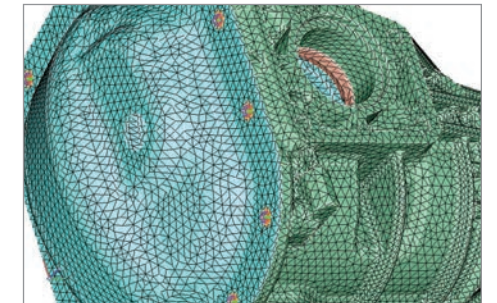
트랜스미션 하우징 메쉬
