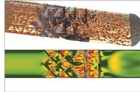
SMX 스타일 믹서 내부의 흐름 패턴 및 속도장 해석
