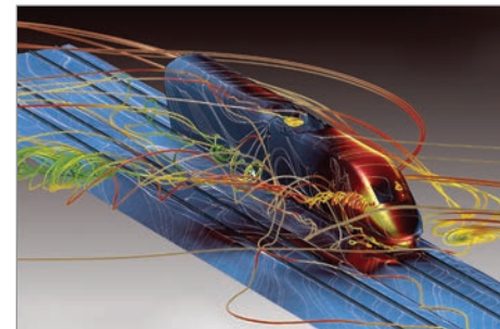
직교류에서의 레일 주위로 나타나는 압력장 및 유선
