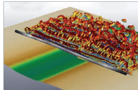
소용돌이의 유동 진동에 의해 발생하는 헤저 파이프 라인의 휘어짐
