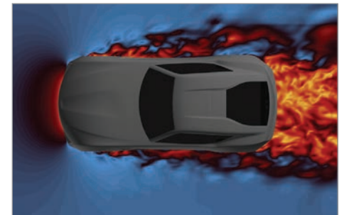
스포츠카의 DES (Detached Eddy Simulation) 흐름
